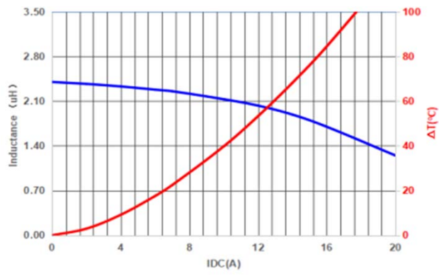
JRPI 0603F-2R2
