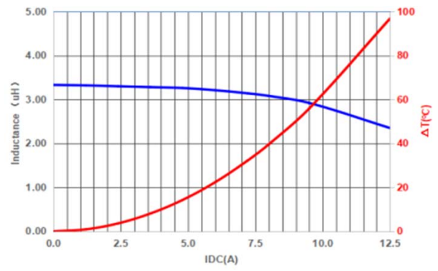
JRPI 0603F-3R3
